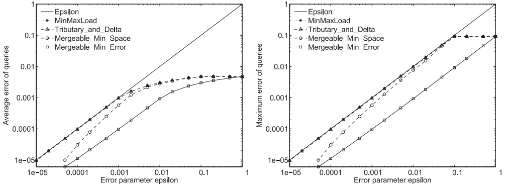
Fig. 3. Heavy hitters: \varepsilon vs. actual error.
