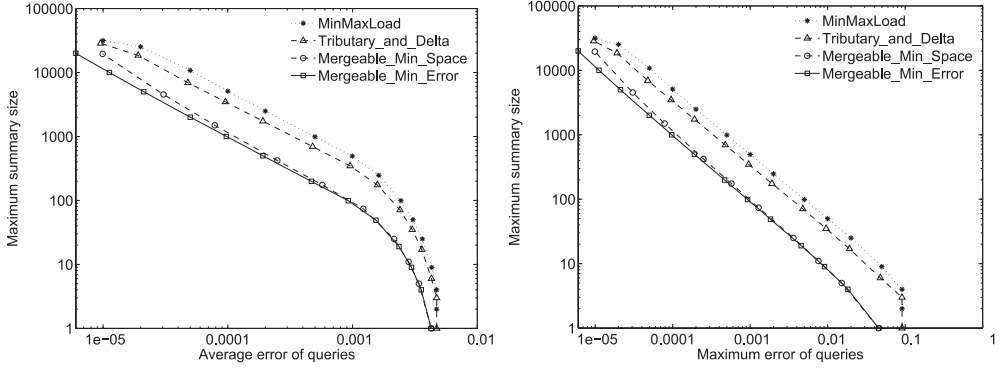
Fig. 4. Heavy hitters: actual error vs. summary size.
