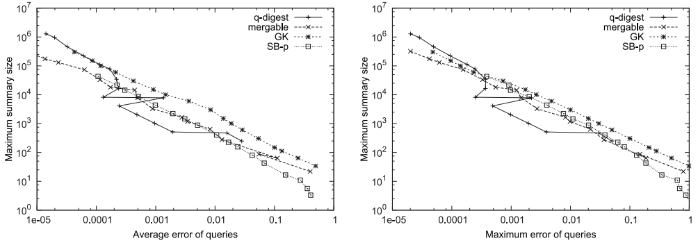
Fig. 5. Quantiles: actual error vs. summary size.
